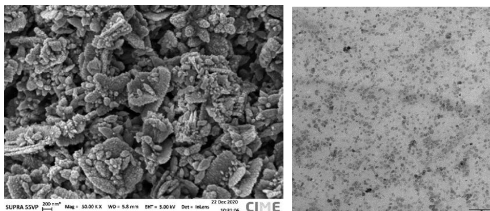
Imagen obtenida por microscopía SEM (izquierda) y TEM (derecha) de las NPs de ZnO
